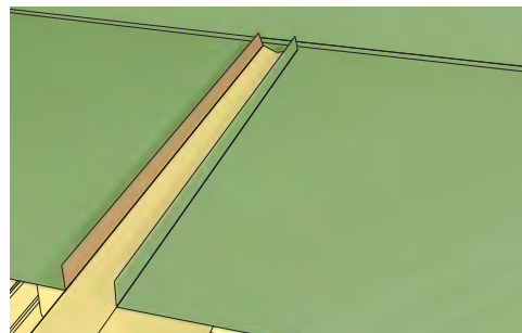
3. Taita viilletyt kohdat ylös kuvan mukaisesti.
