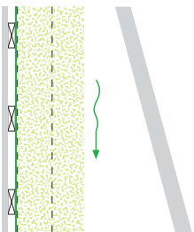
Yläpohja puhalluseristeillä
