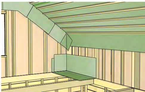
1. Taita puolet ilman/höyrynsulusta sivuseinää vasten ja puolet kattoristikoiden päälle. Jätä sulkua päätyseinälle noin 500 mm.
