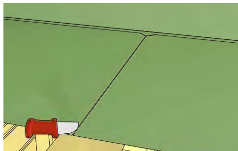
2. Viillä ilman/höyrynsulun taitteeseen kuvan mukainen kolmio ristikon alapaarteen kohdalle. Jatka viiltoa alapaarteen keskikohtaa pitkin.
