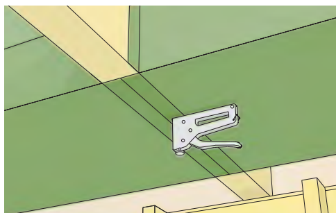
10. Kiinnitä ilman/höyrynsulku ristikon alapintaan nitojalla.
