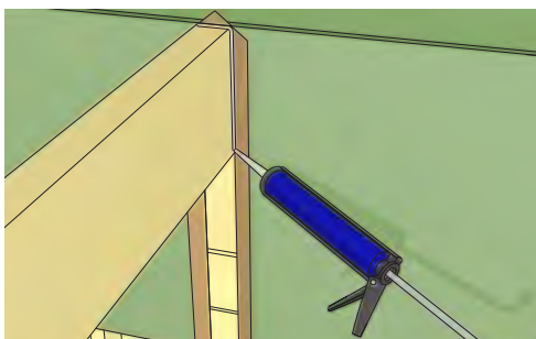
5. Taita ilman/höyrynsulun osat pois edestä ja pursota tiivistemassaa alapaarteisiin.
