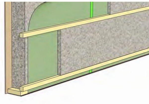
6. Asenna seinän ilmansulun sisäpuolelle vaakakoolaus ja vaakaeiste rakennesuunnitelmien mukaan. Vaakakoolaus pitää ilmansulkujen limitykset yhdessä ja luo tilan myös sähköasennuksille, jolloin ilmansulku pysyy ehyenä.
