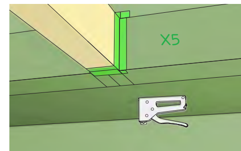
12. Lisää seuraava ilman/höyrynsulku kattoristikoiden alapintaan. Limitä seinän sulun kanssa n. 500 mm.
