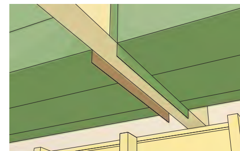
8. Käännä Ilman/höyrynsulku katon suuntaiseksi.
