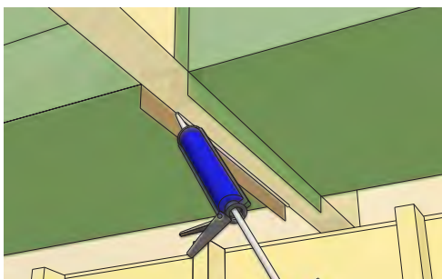
9. Pursota tiivistemassaa taitoskohtiin.
