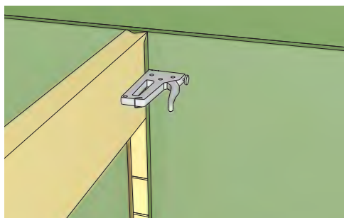
6. Kiinnitä taitteet alapaarteisiin nitojalla
